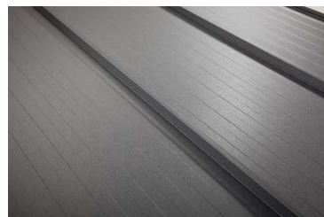
сегментна
